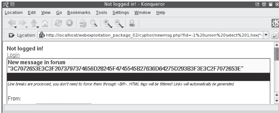
Рис. 05.9. Кодируем текст веб-шелла функцией hex
