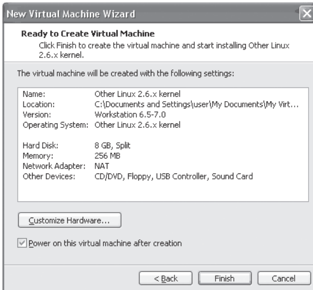
Рис. 02.6. Мастер создания виртуальных машин, шаг 5
