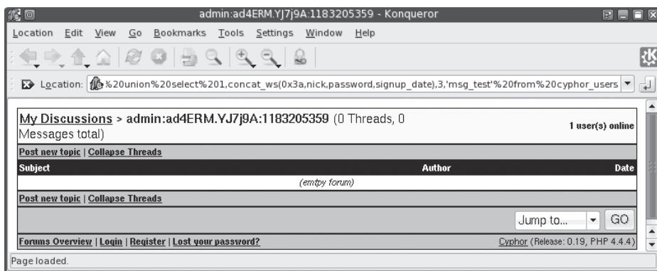
Рис. ПЗ.1. Извлекаем из базы имя пользователя, хэш пароля и время создания (в секундах)
