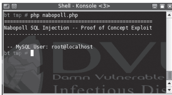
Рис. 07.5. Работа эксплойта для NaboPoll
