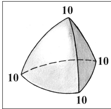
Рис.5. Сферотетраэдр (сфетраэдр) как форма кристалла орихалка: плод пересечения сфер, помещенных в вершины тетраэдра и радиусом равных его ребру
