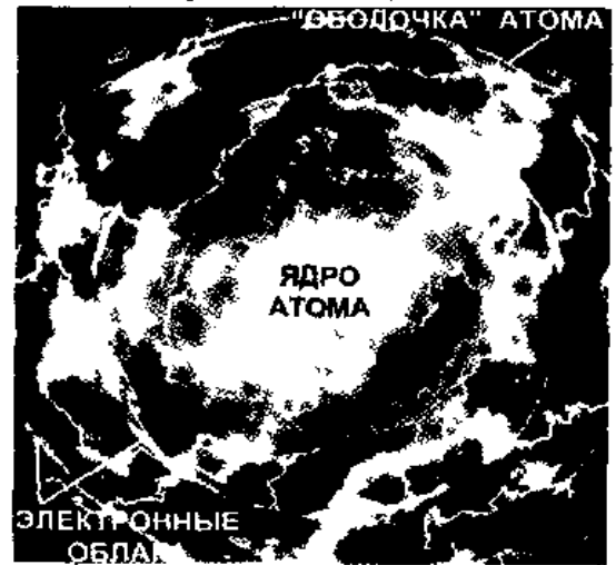
Рис. 1.4-9 Б. Электронная структура атома гелия по данным [32]
