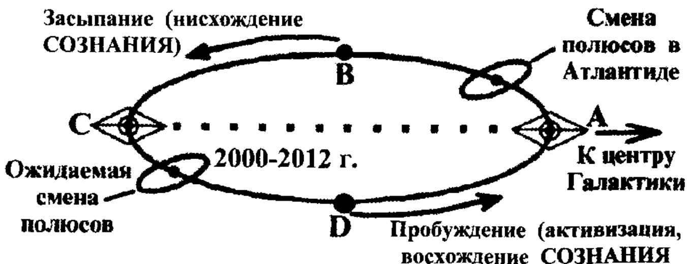
Рис. 1.0-1. Схема цикла прецессии равноденствий [2].
