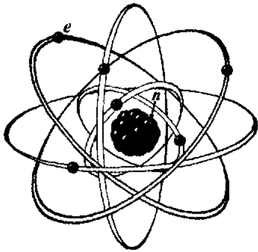
Рис. 1.6-4 А. Модель атома – схема ДУШИ на уровне атомов
