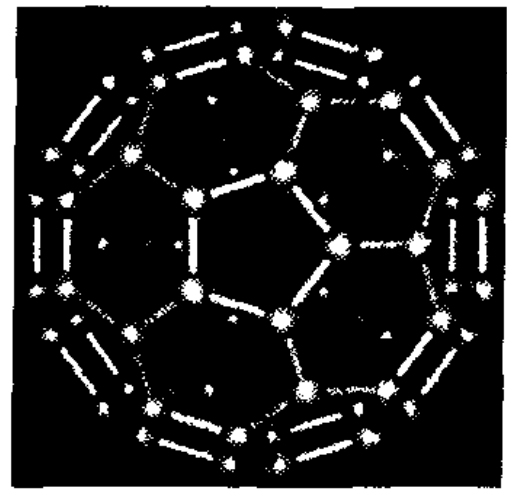
Рис. 1.6-4 Б. Модель фуллерена (C 60 ) – схема ДУШИ на уровне молекул
