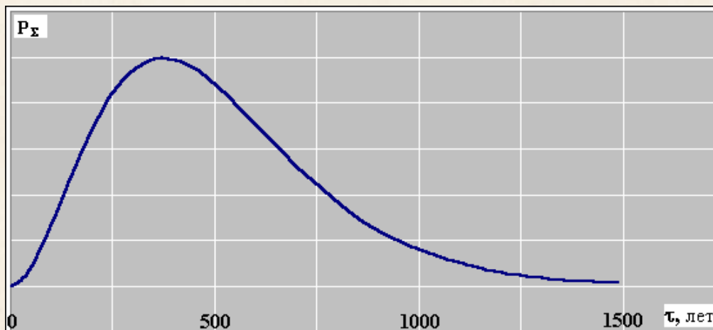
Рис. 1. Зависимость пассионарной энергии этносистемы во времени P_{\Sigma} = P_{\Sigma}(t)
